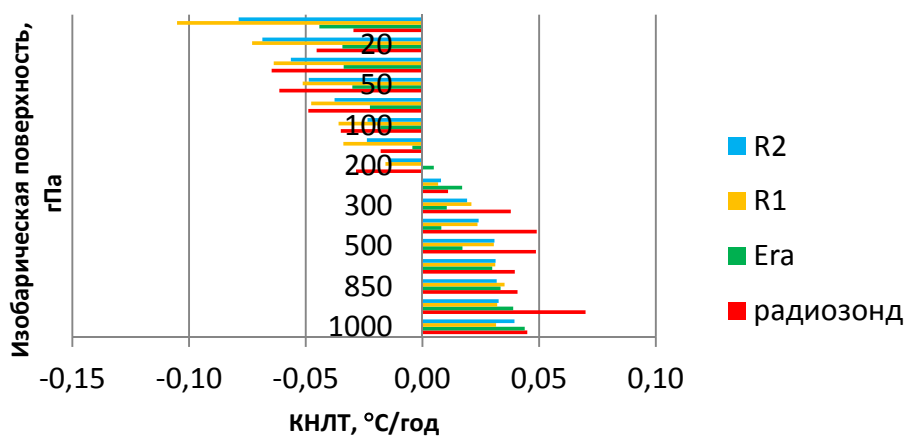
Рис.1. Коэффициент наклона линейного тренда среднегодовых значений температуры тропосферы и нижней стратосферы для станции Казань
