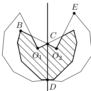
Рис. 3. Пересечение двух кругов с вырезанными секторами. Здесь \angle O_1O_2B = \angle O_2O_1C — угол поворота, \angle BO_2E — угол вырезанного сектора, |O_1O_2| — расстояние между центрами, прямая CD — прямая отражения пересекаемых кругов с вырезанными секторами относительно друг друга
